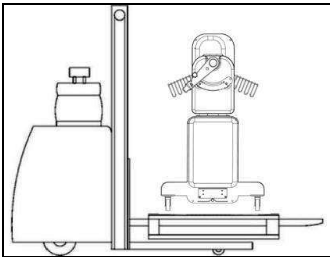
SFG 500 T - 500 TM
